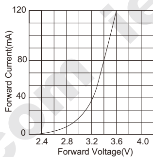
Fig.1 正向电流 Vs. 正向电压
