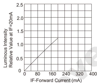
Fig.2 相对亮度 Vs. 正向电流
